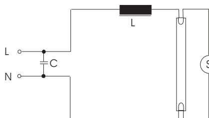
Induktive Schaltung
