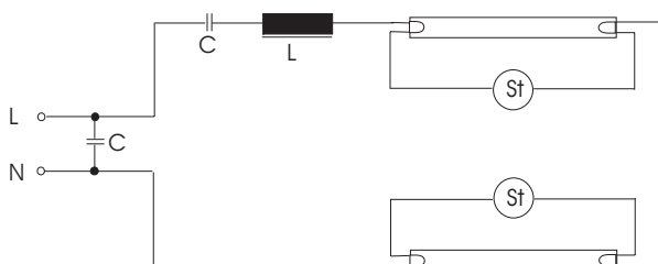
Kapazitive Tandemschaltung
