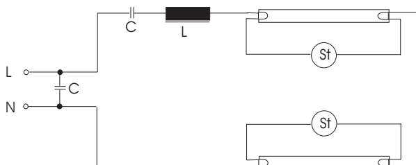
Kapazitive Tandemschaltung
