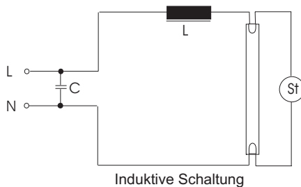
Induktive Schaltung
