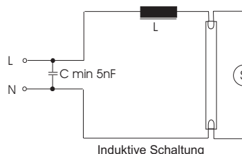
Induktive Schaltung
